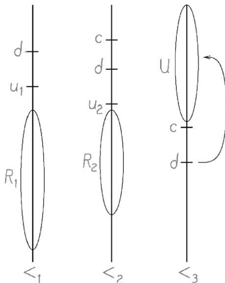
Fig. 1. The orders <_1 , <_2 and <_3 .
